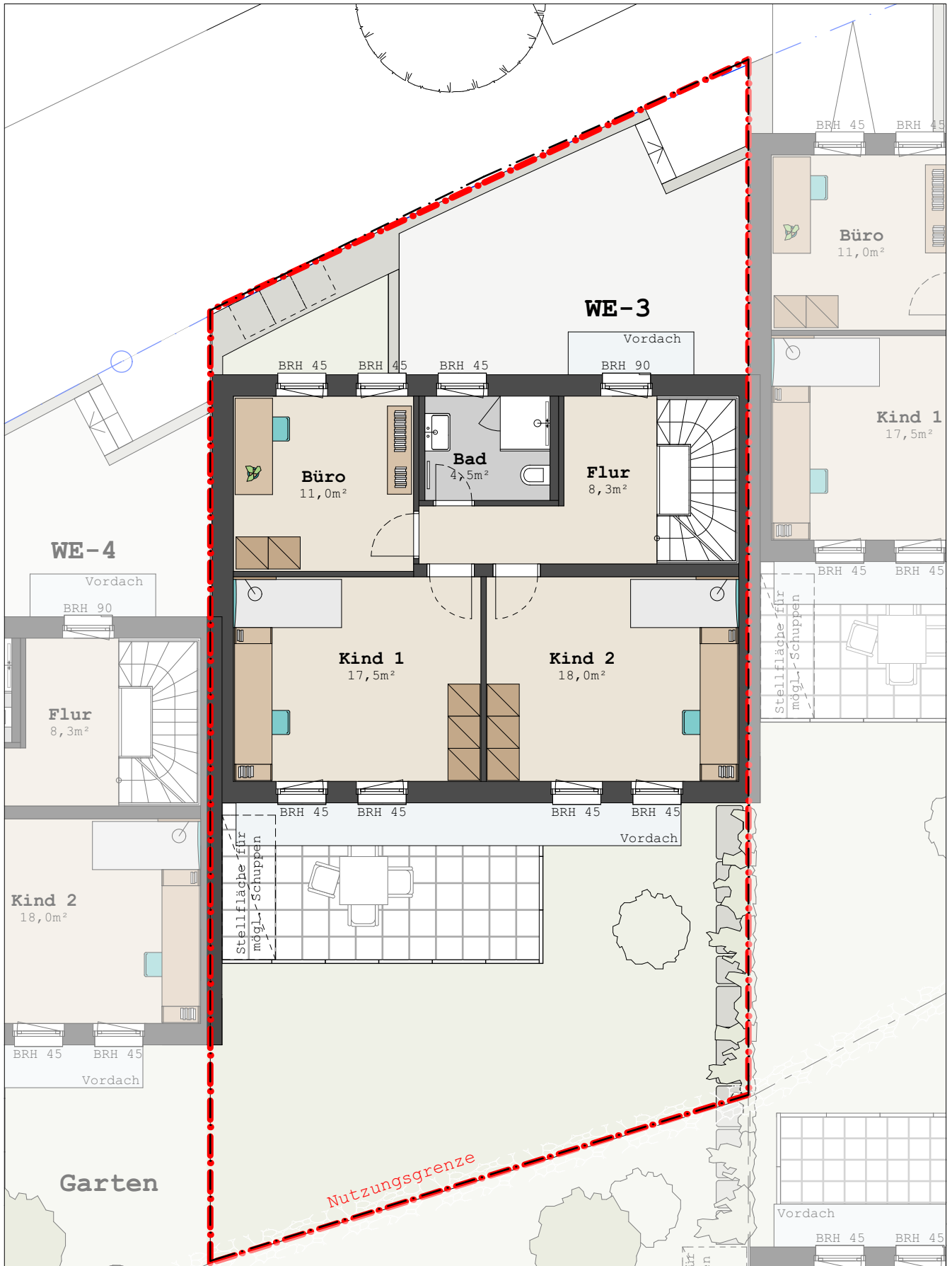
WE-3 | Mittelhaus | Stand 29.09.2017 Obergeschoss M 1:100 A4
