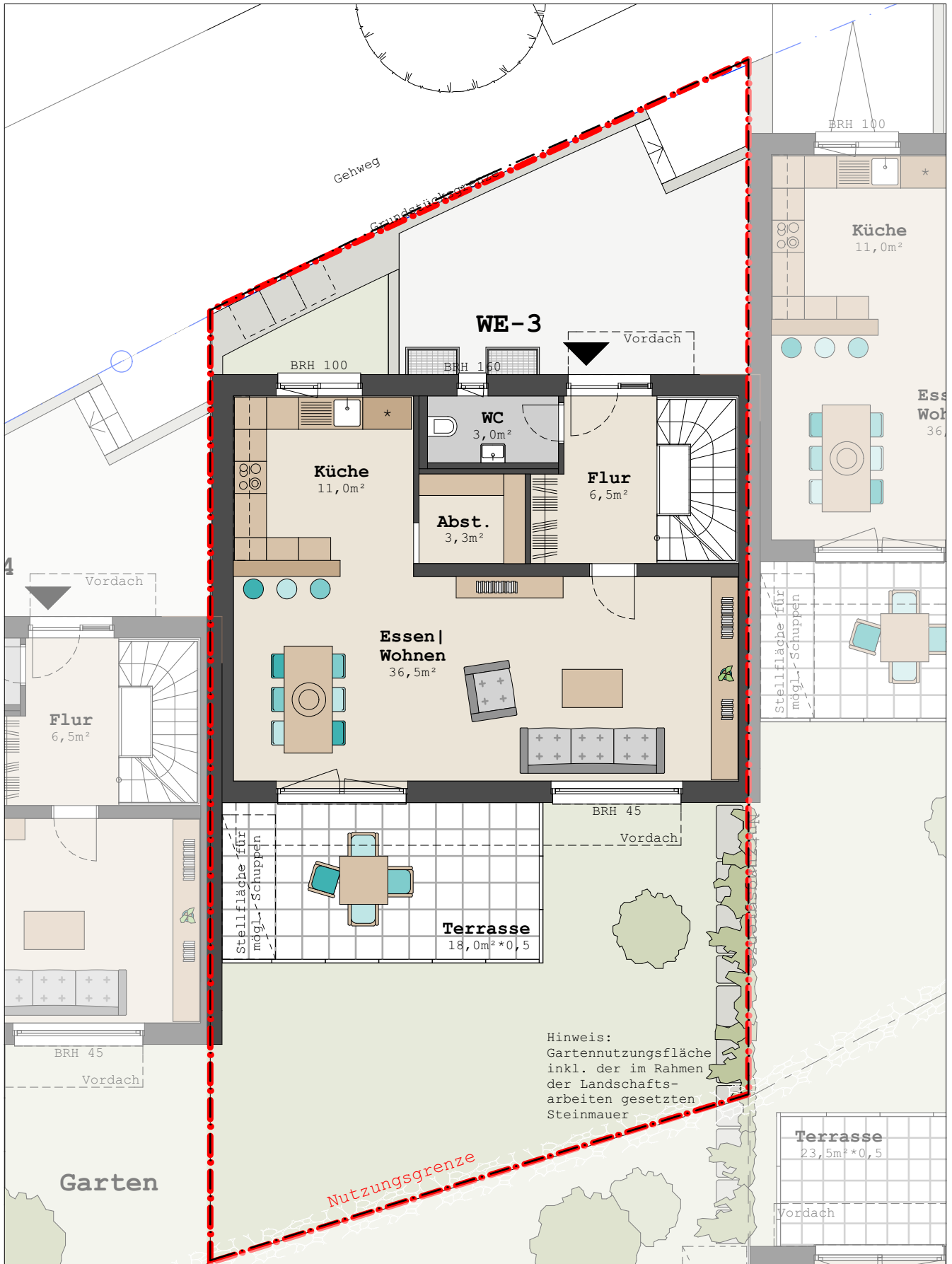
WE-3 | Mittelhaus | Stand 29.09.2017 Erdgeschoss Variante offene Küche M 1:100 A4
